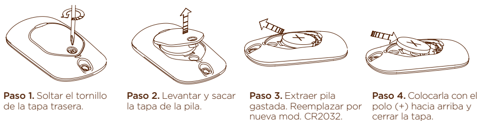
Fig. 2 Sustitución de la batería.
