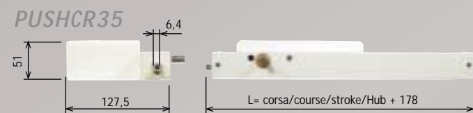
Gruppo trasmissione di potenza per PUSH CR35 Groupe de transmission de puissance pour PUSH CR35 Drive assembly for PUSH CR35 Leistungsübertragung für PUSH CR35
