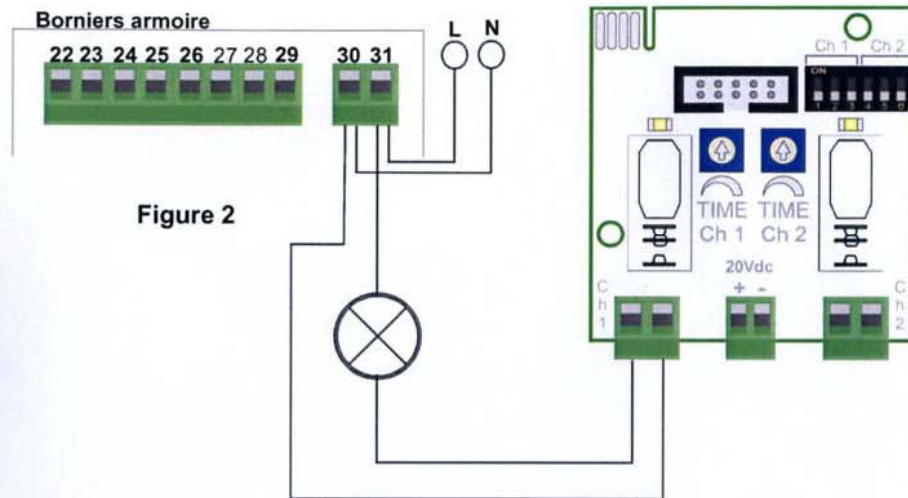
Borniers armoire
